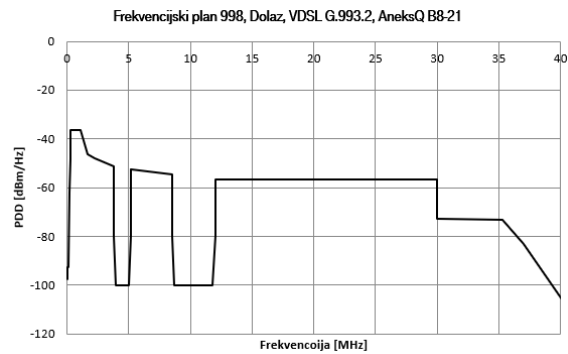
Slika 5.6.1 Frekvencijski predložak za VDSL2 frekvencijski plan 998, B8-21 dolaz (crno).
