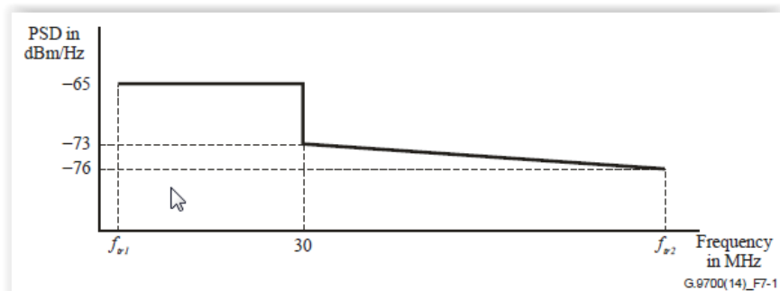
Slika 4.9.1 - Maska PSD za G.fast 106 MHz profil
