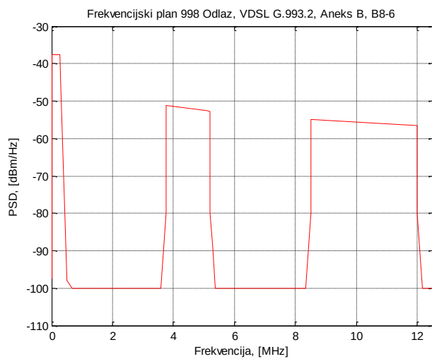
Slika 5.7.2 Frekvencijski predložak za odlazni smjer prijenosa za VDSL2, frekvencijski plan 998, B8-6
