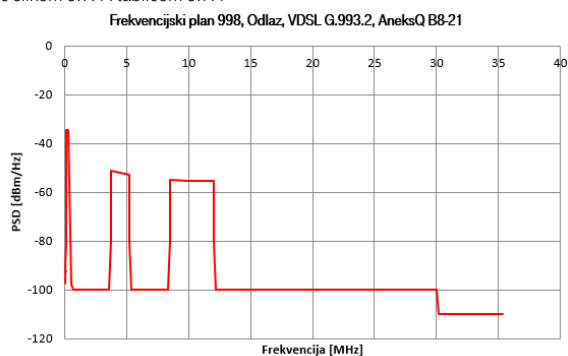
Slika 5.7.4 Frekventijski predložak za odlazni smjer prijenosa za VDSL2, frekventijski plan 998, B8-21
