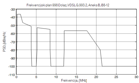
Slika 4.8.4 Maska PSD za VDSL2 frekvencijski plan 998, B8-12 dolaz (crno).
