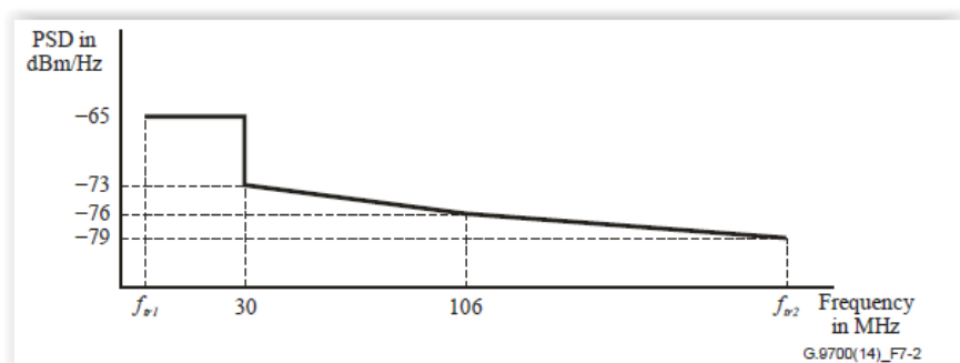
Slika 4.9.2 - Maska PSD za G.fast 212 MHz profil*
