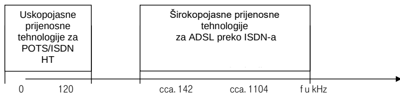
Slika 1. Frekventijski opseg za uskopojasne i širokopojasne prijenosne tehnologije
